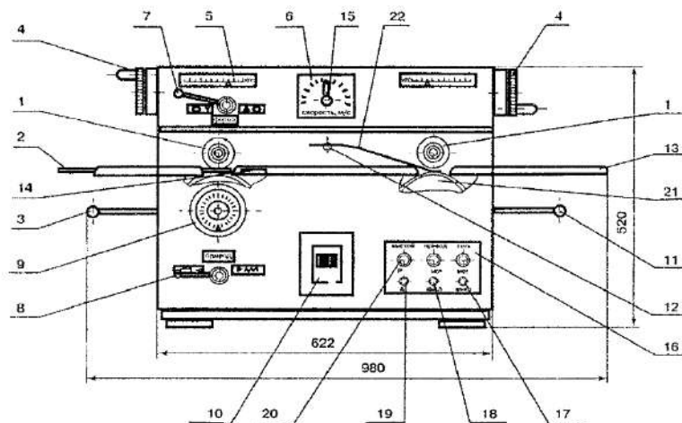
Схема прободрукарського пристрою ЛПУ-1:
